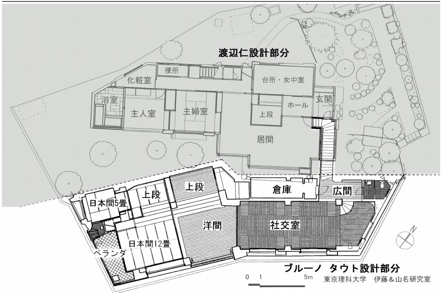
① 旧日向家熱海別邸平面
