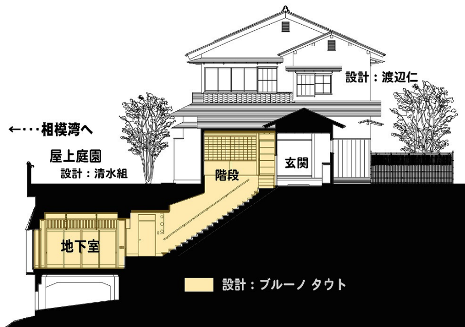
② 旧日向家熱海別邸断面
